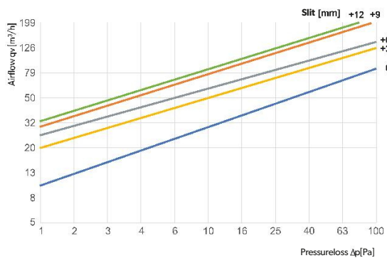
ASV160-ML - levegő elszívás
