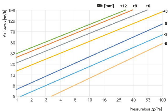
ASV150-ML - levegő befűvés
