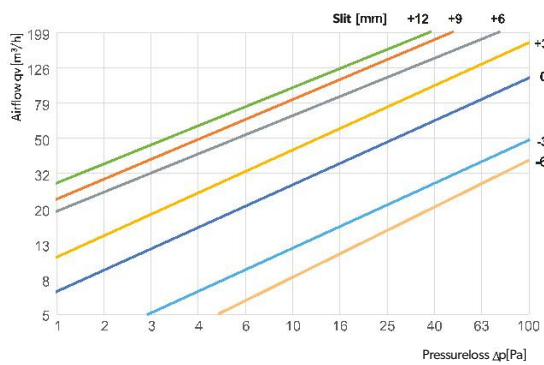
ASV150-ML - levegő elszívás
