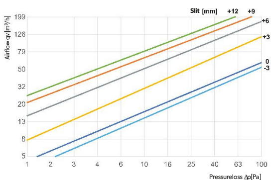
ASV125-ML - levegő befűvés
