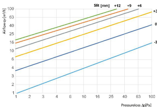
ASV100-ML – levegő befűvés
