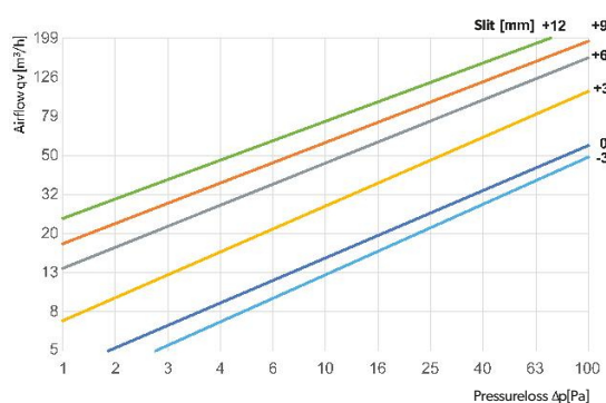
ASV125-ML - levegő elszívás
