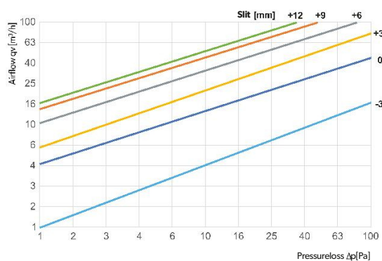
ASV100-ML – levegő elszívás
