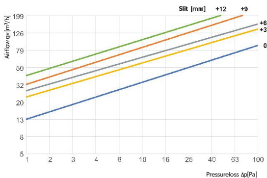
ASV160-ML - levegő befűvés
