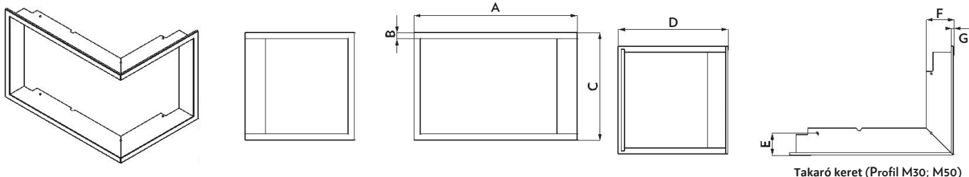
Takaró keret (Profil M30; M50)
